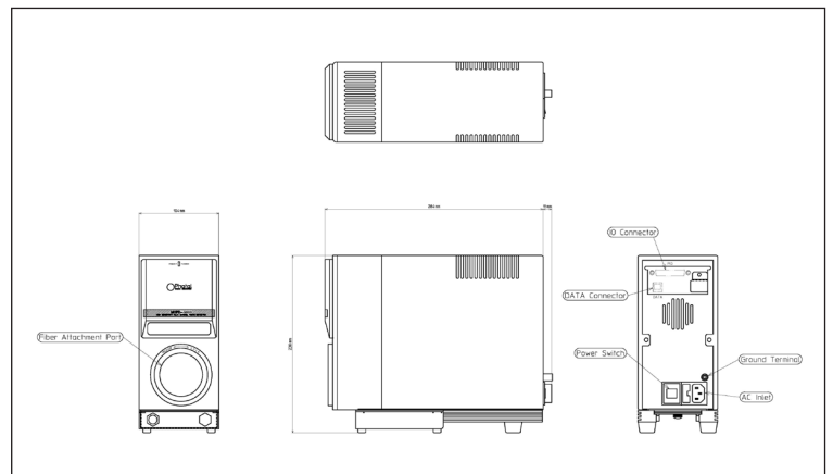
CDS-30x0 Dimensions
